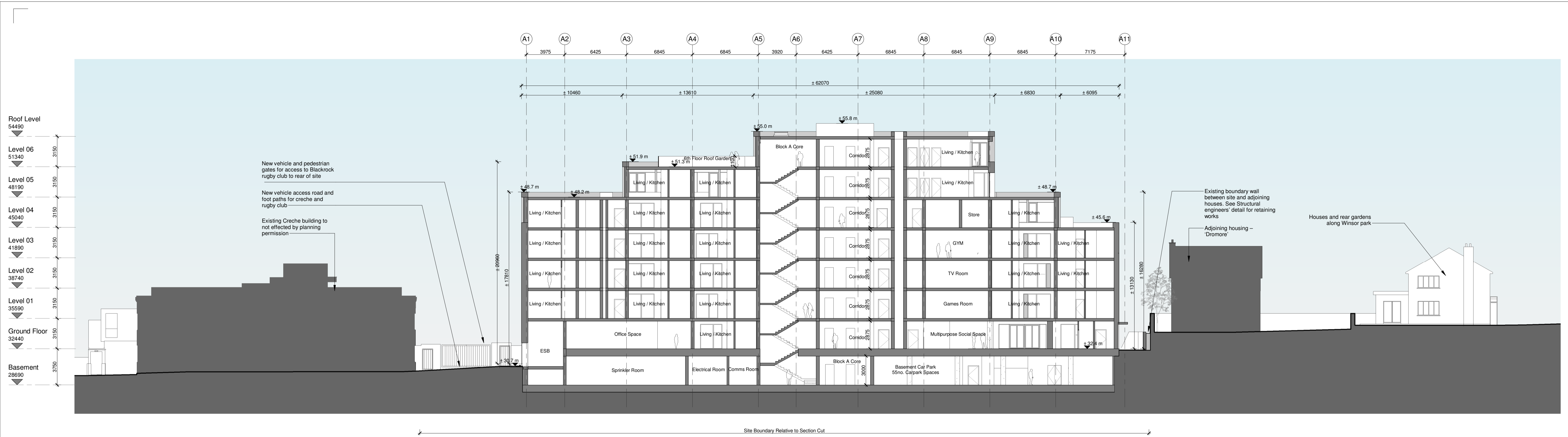
1 Section A-A scale 1 : 200
